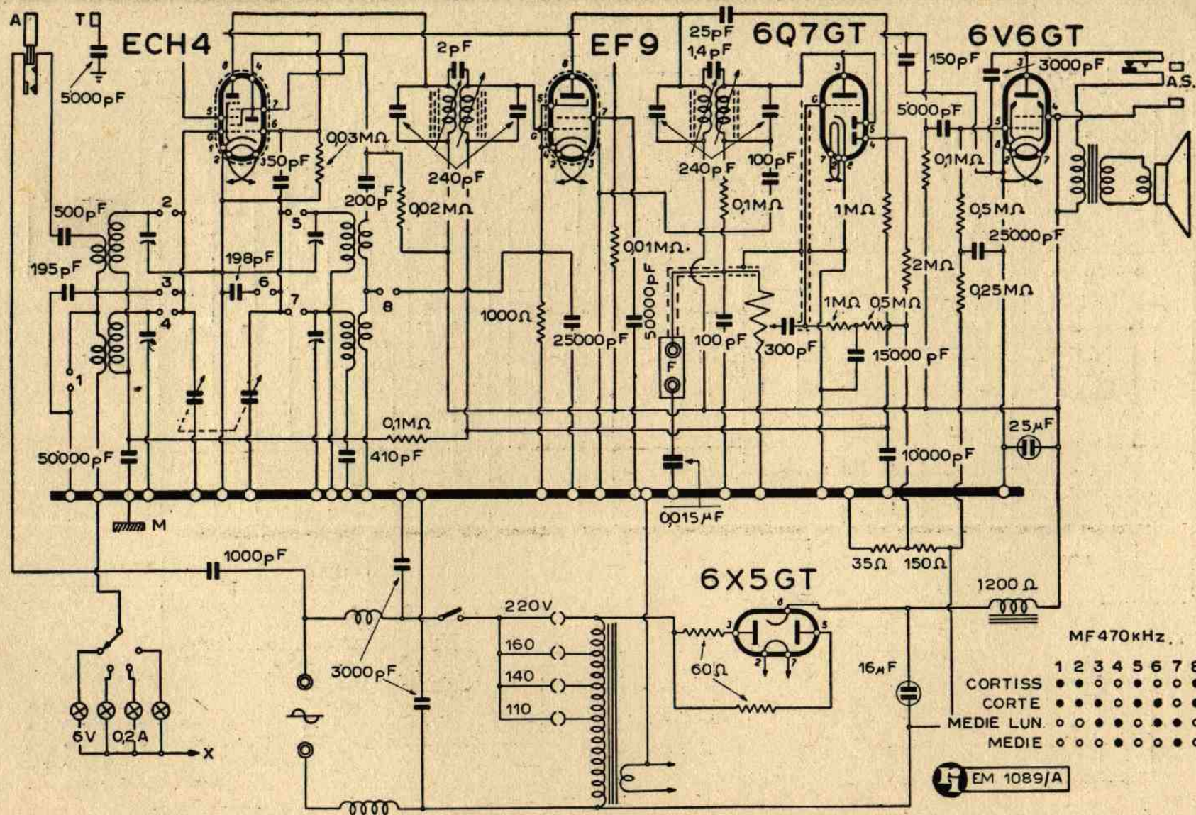
Lo schema elettrico del Phonola 577-A
